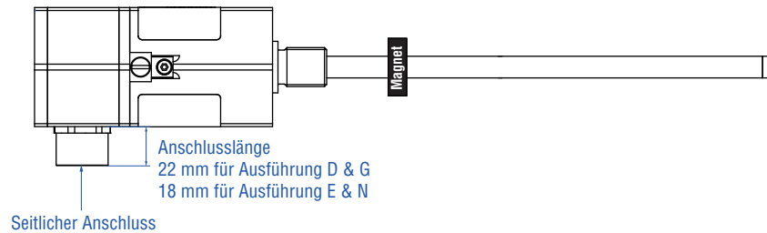
Seitlicher Anschluss
