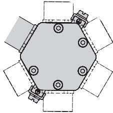
C01/N01: Stecker auf 6 verschiedenen Positionen, jeweils bei 60°
